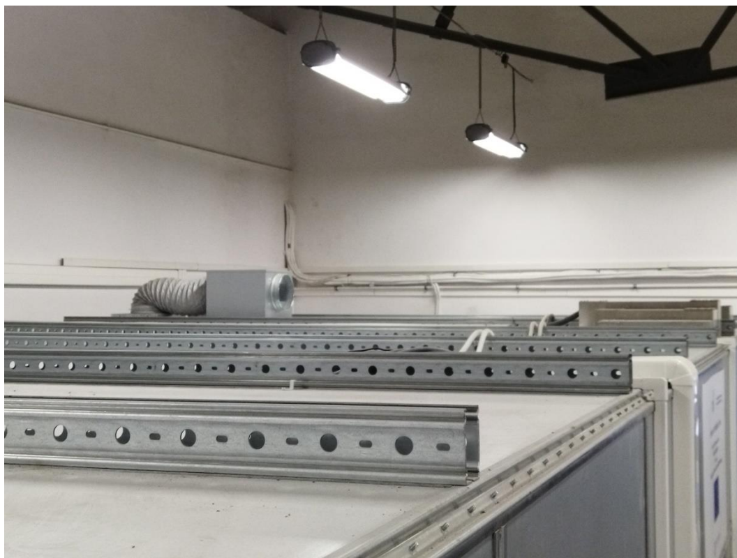
IMG_20211213_091040 Strop komory rewerberacyjnej – widok na prowadnice kablowe i układ filtrowentylacji w przedniej części komory
